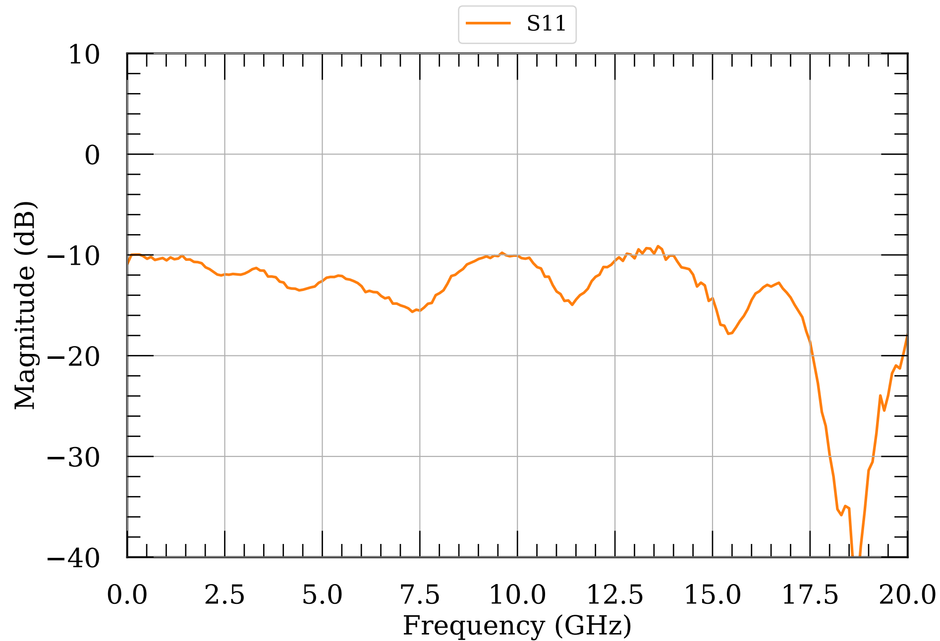
LNA S-params module042
